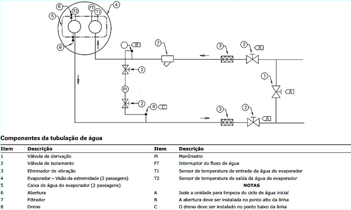
Figura 1 – Diagrama típico de tubulação
